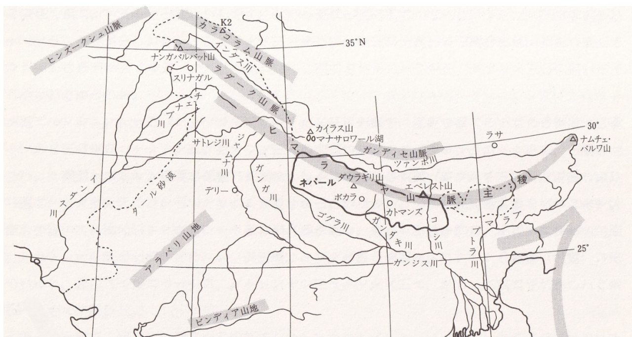
ヒマラヤ概念図：在田一則『ヒマラヤはなぜ高い』より
